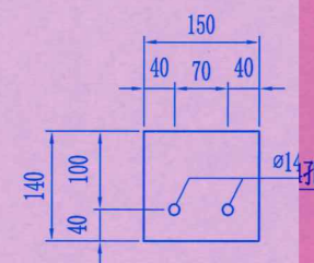
①大样
